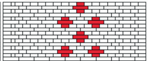
Bild 2 Kreuzverband
