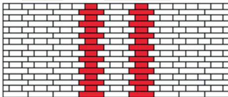
Bild 1 Blockverband
